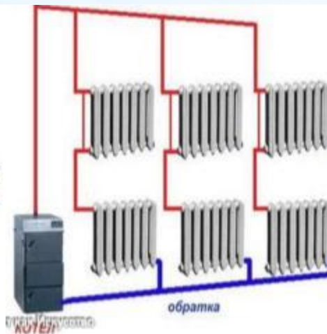
Система отопления
